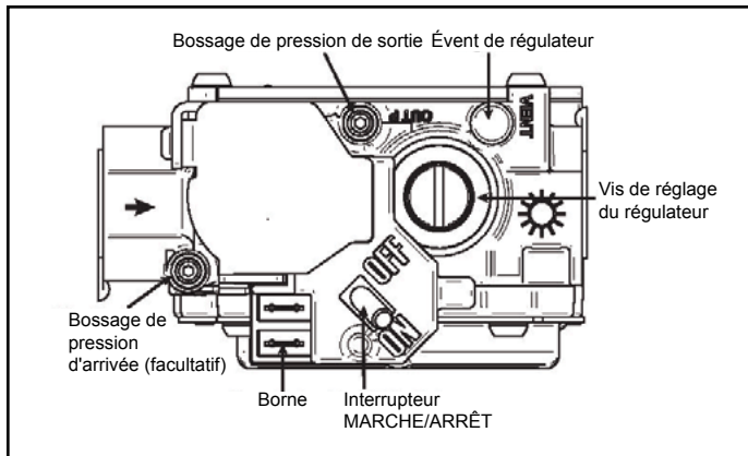
FIG. 28. - SOUPAPE DE GAZ WHITE RODGERS 36J24-214
