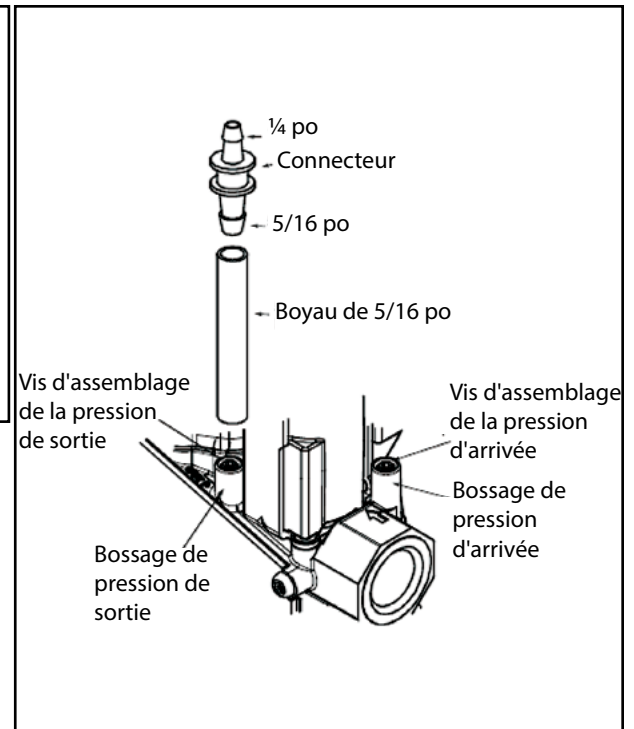
FIG. 29. TROUSSE DE VÉRIFICATION DE LA PRESSION DE LA SOUPAPE
